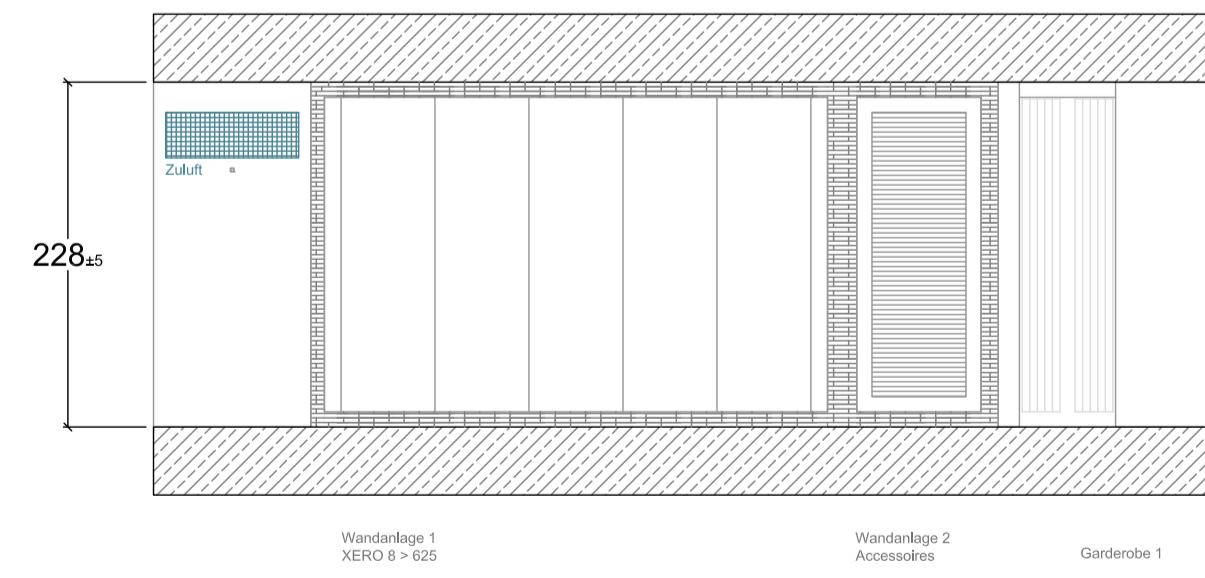
Wandansicht UG 3
